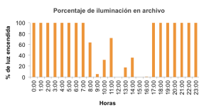
Gráfico 10. Ejemplo de resultado gráfico obtenido con un registrador de ocupación.
