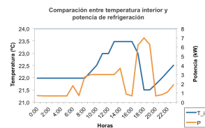
Gráfico 9. Ejemplo de resultado gráfico obtenido con un registrador de temperatura.
