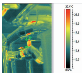
Figura 30. Termografía a las tuberías de una bomba de calor.
