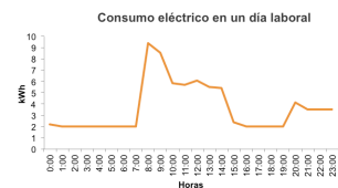
Gráfico 8. Ejemplo de resultado gráfico obtenido con un analizador de redes en una oficina.
