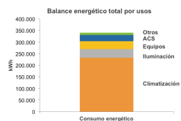
Gráfico 6. Ejemplo de balance energético total por usos.
